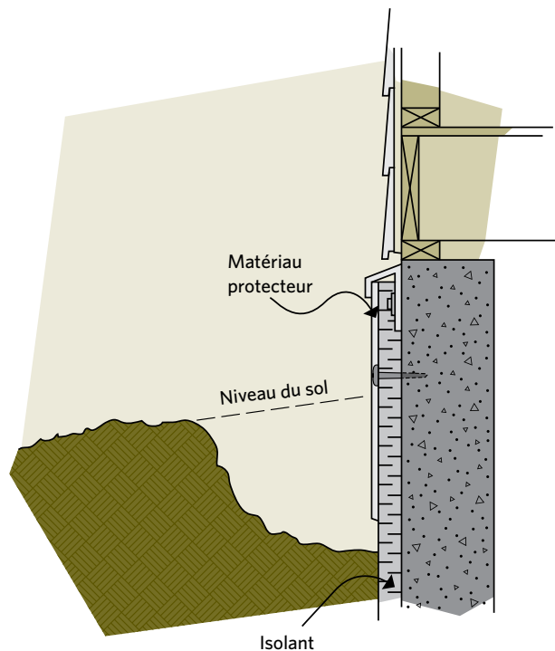
Figure 6-9 La protection extérieure doit s'étendre sous le niveau du sol
