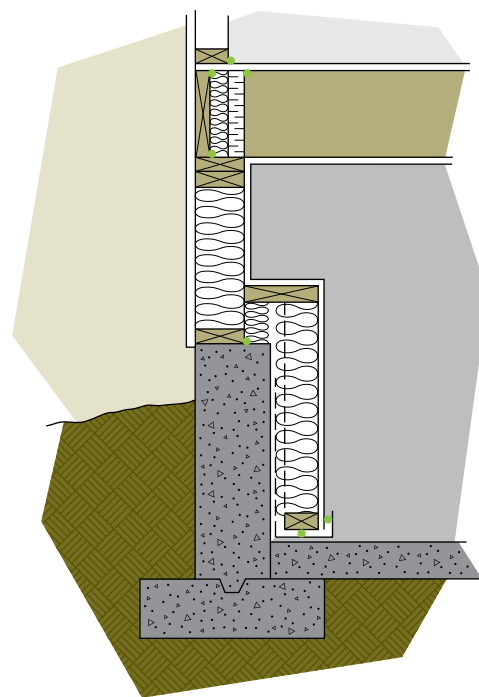
Figure 6-20 L'isolation d'un mur bas se fait en deux étapes et forme une pièce d'appui
