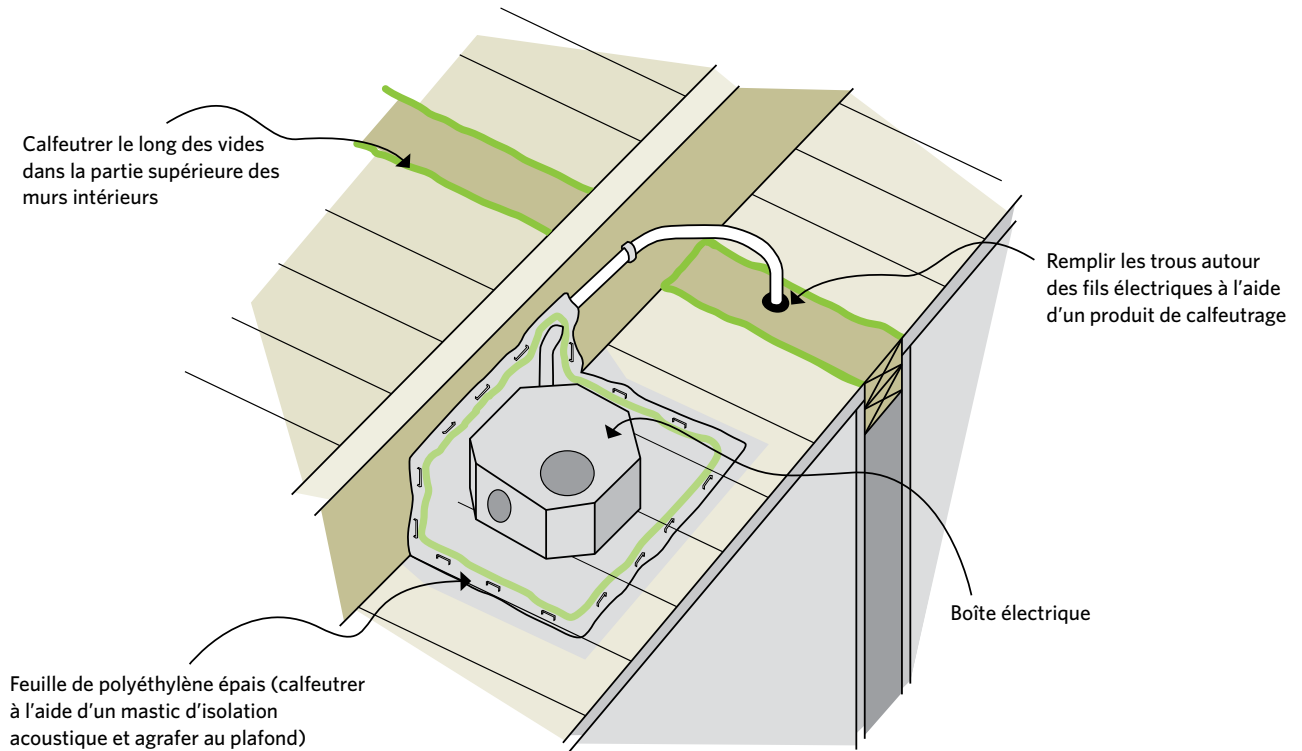
Figure 5-8 Sceller un luminaire au plafond
