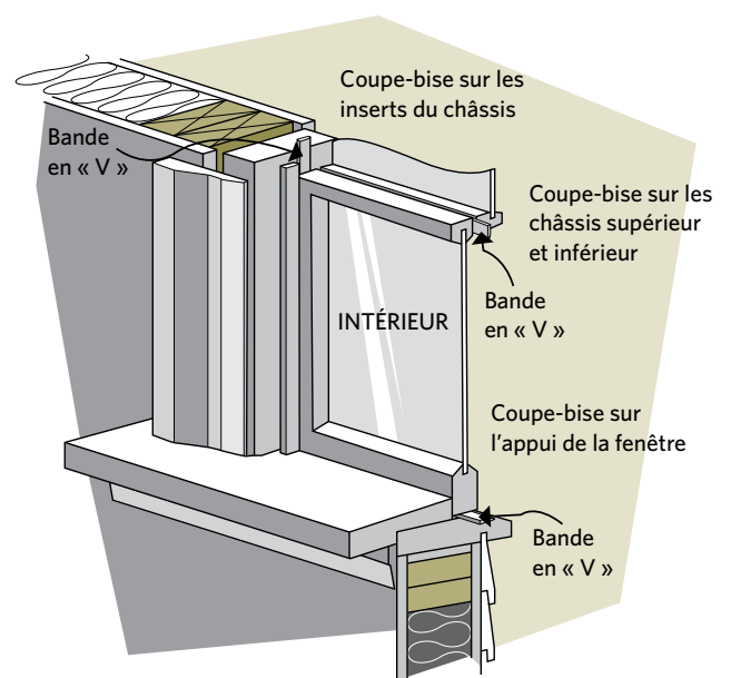
Figure 8-5 Où installer les coupe-bise sur une fenêtre à guillotine
