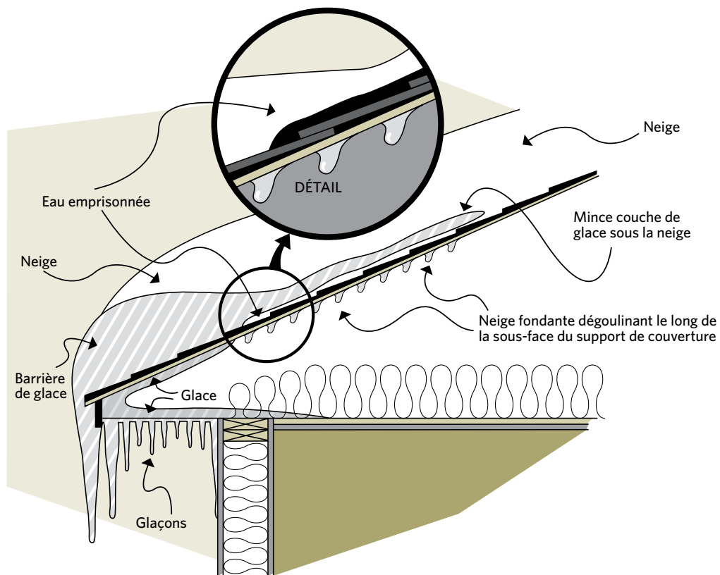
Figure 5-21 Barrières de glace
