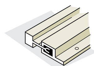
Coupe-bise par effet de ressort
