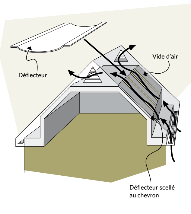
Figure 5-19 La ventilation se fait entre les sections grâce aux événements d'entretoit installés entre les chevrons
