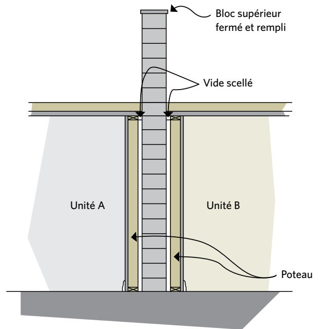
Figure 7-3 Construction en blocs de béton, un mur mitoyen et un mur ouvert
