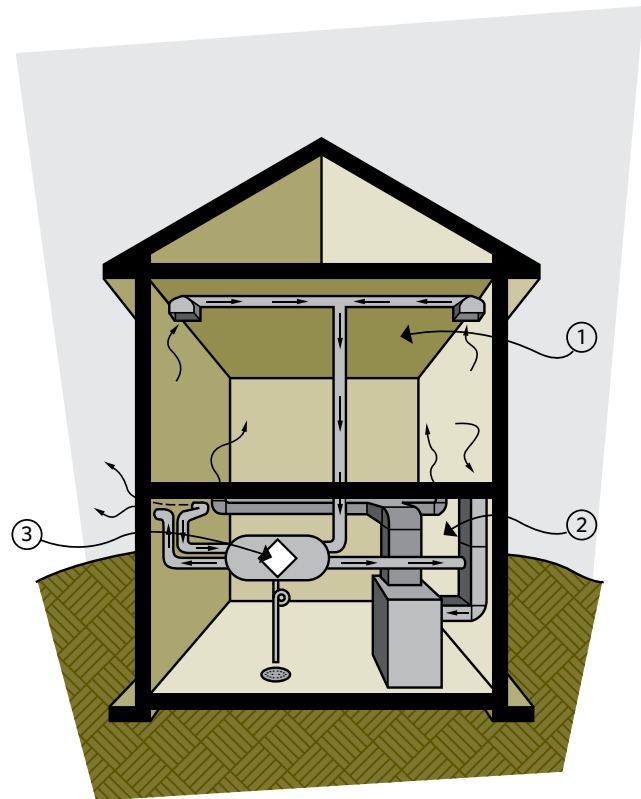
Figure 9-3 Ventilation d'une maison au moyen d'un ventilateur-récupérateur de chaleur
