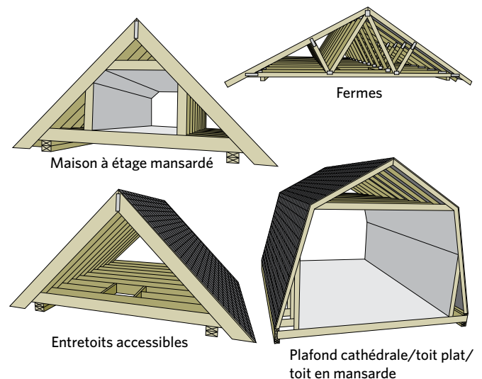
Figure 5-1 Types d'entretoits
