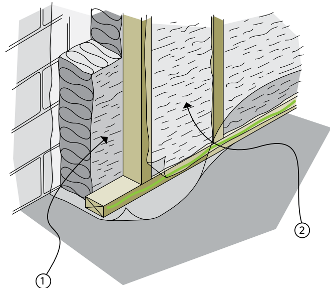
Figure 6-14 Double couche de matelas isolant dans un mur à ossature
