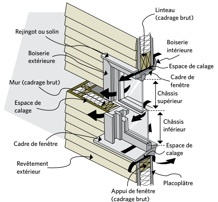
Figure 8-2 Vue en coupe d'une fenêtre à guillotine double montrant les pièces et les endroits où il y a des fuites d'air
