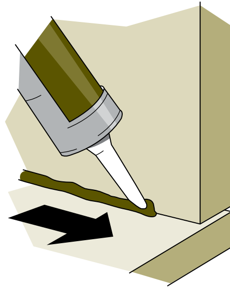
Figure 4-4 Comment étendre un cordon de pâte à calfeutrer
