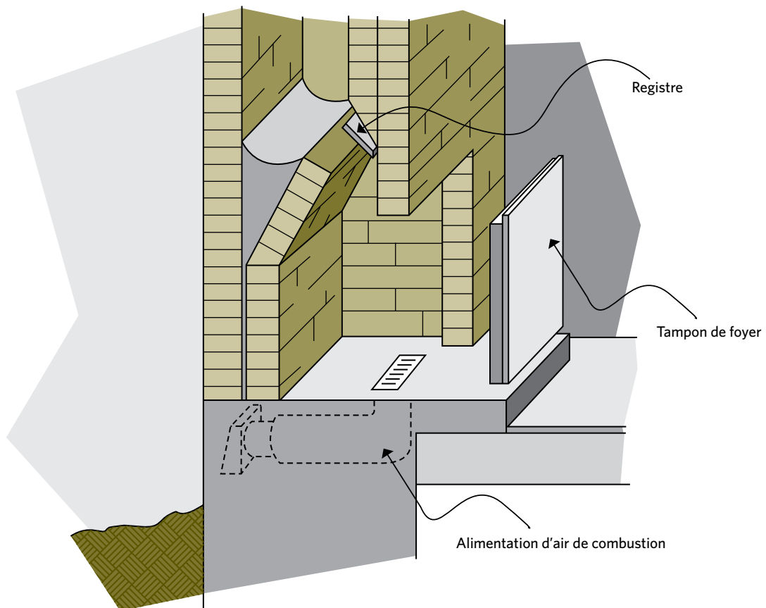
Figure 4-6 Conduit pour l'air de combustion extérieur pour alimenter le foyer
