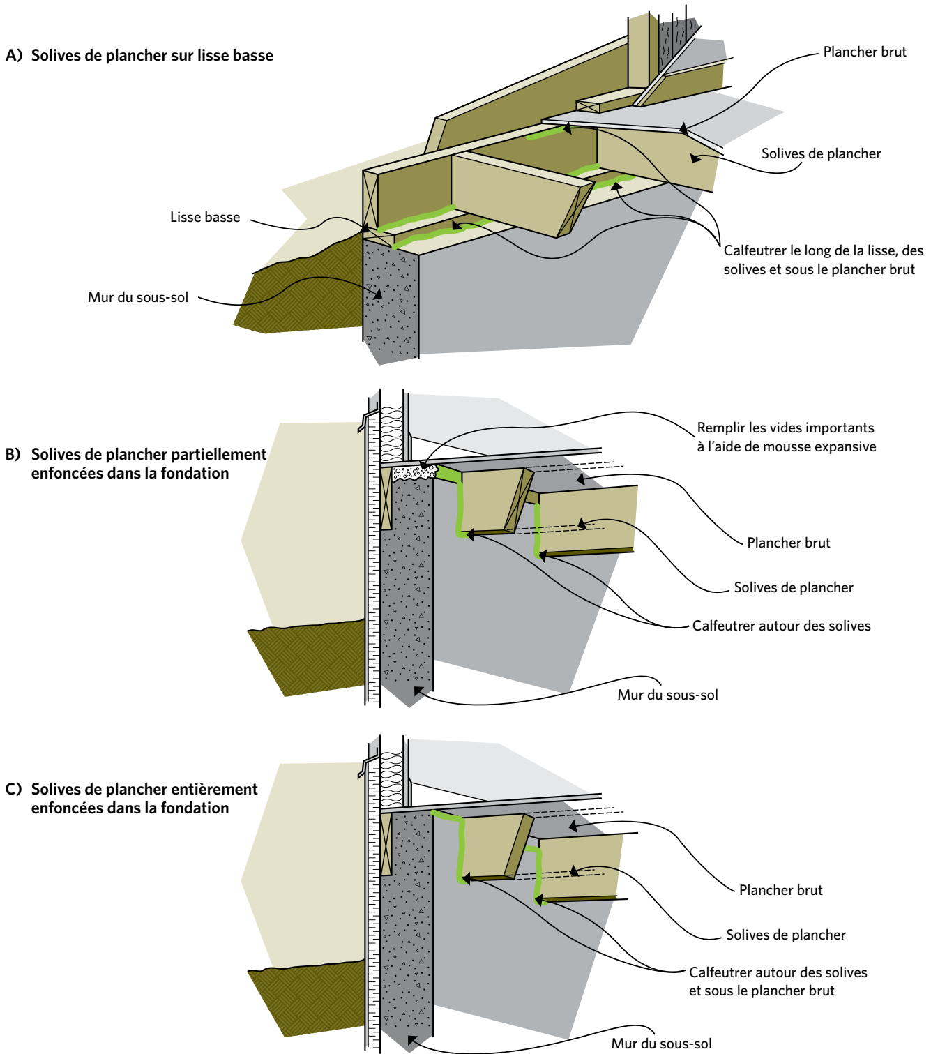
Figure 6-18 Réduction des fuites d'air dans l'espace entre les solives
