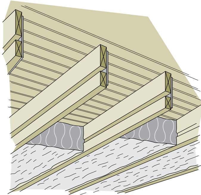
Figure 5-24 En rallongeant les chevrons, on a plus d'espace pour l'isolant et la ventilation
