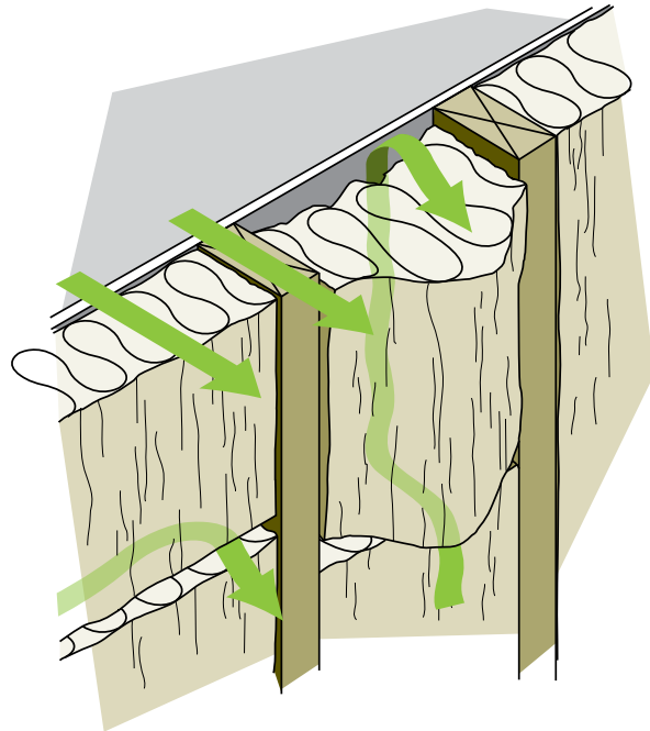
Figure 2-5 Pont thermique et courants de convection dans une cavité murale
