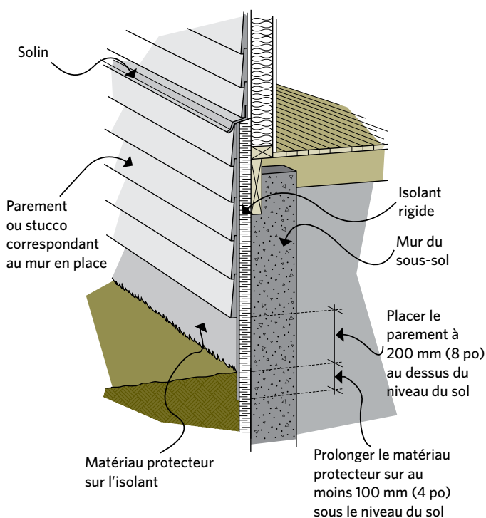
Figure 6-8 Isolation de la solive de bordure de l'extérieur
