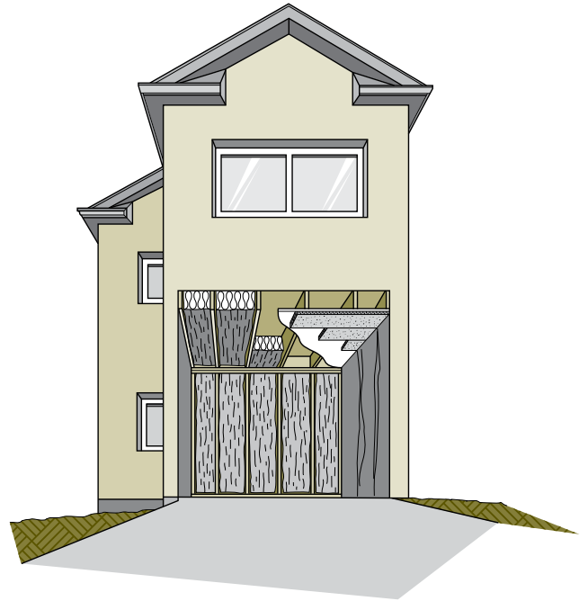
Figure 7-11 Étanchéisation et isolation entre la maison et un garage non chauffé
