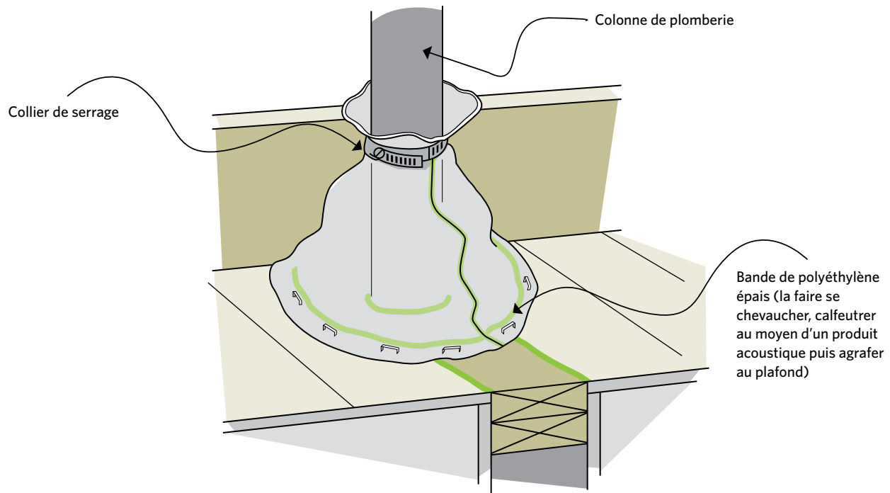
Figure 5-6 Sceller la colonne de plomberie
